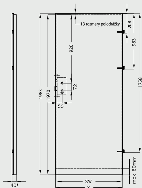
Křídlo s polodrážkou
