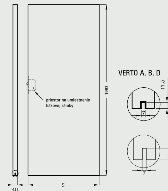
Křídlo bez polodrážky
