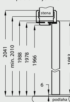
vyžadovaná výška otvoru ve zdi 2010 mm
