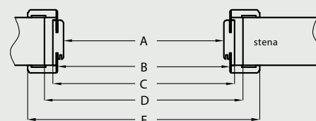
D - vyžadovaná šířka otvoru ve zdi
